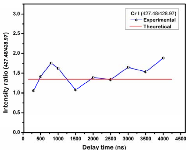
شکل ۵. تحول زمانی نسبت شدت دو خط Cr I ۴۲۷/۴۸ nm و ۴۲۸/۹۷ به همراه نسبت شدت تئوری آن‌ها (خط مستقیم)
