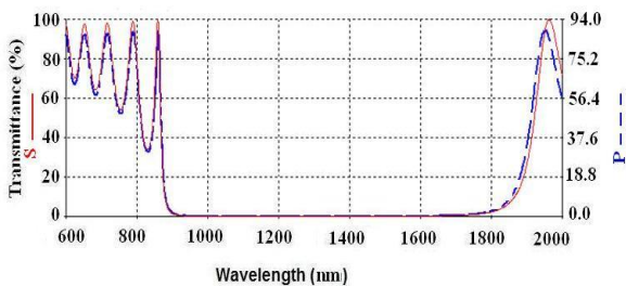
شکل ۵. محاسبات طیف عبوری از بلور فوتونیک شبه فلز - دی‌الکتریک برای قطبیدگی‌های S, P، N=10 ، \theta=10^\circ .
