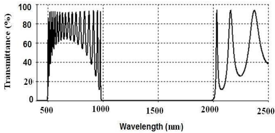
شکل ۴. محاسبات طیف عبوری از بلور فوتونیک شبه فلز - دی‌الکتریک با N=10 ، \theta=0^\circ .
